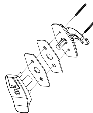
① 不鏽鋼指示門鎖詳圖
