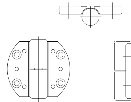
② 不鏽鋼鉸鍊詳圖
