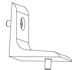
③ 不鏽鋼L型固定座詳圖
