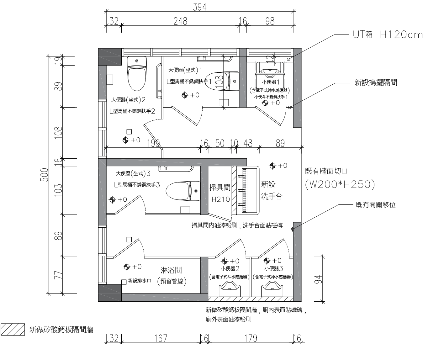
整修平面圖 S:1/50
