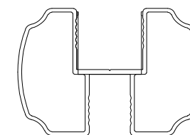
④ 不鏽鋼拉桿詳圖
