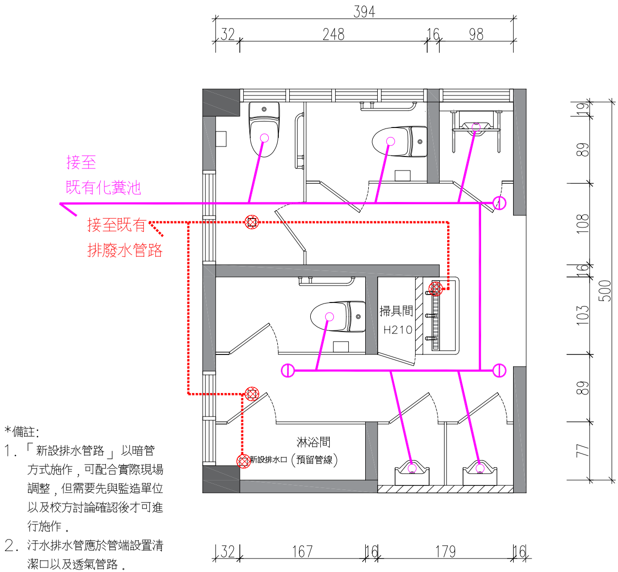
排水平面圖 S:1/50
