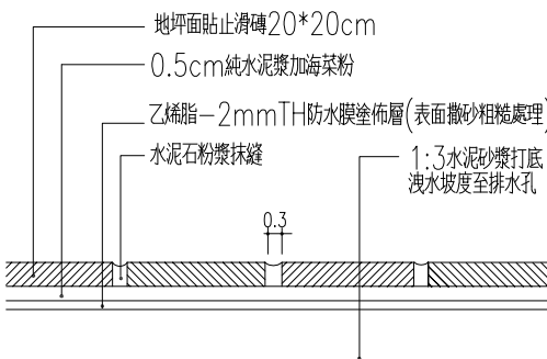
廁所地磚大樣圖
