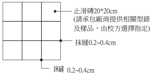
廁所地磚大樣圖
