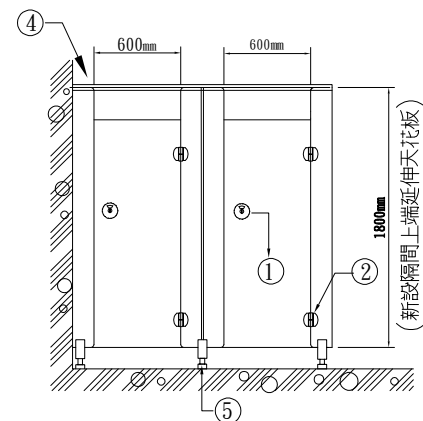
淋浴間隔間（內，外開）正立面圖
