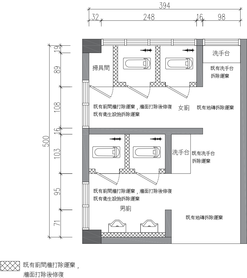
現況平面圖 S:1/50
