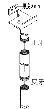
⑤ 不鏽鋼腳座詳圖
