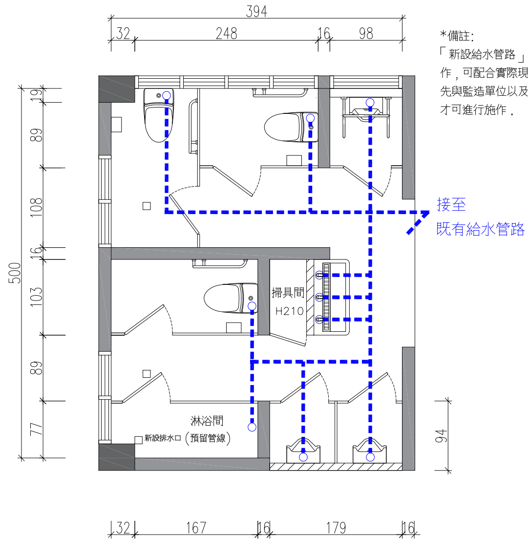
給水平面圖 S:1/50
