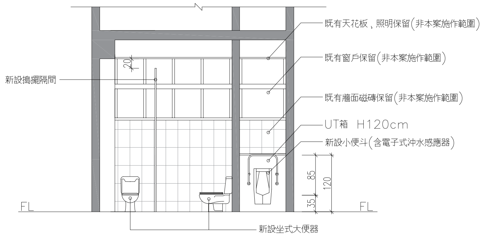
A-A' 剖立面圖 S:1/50
